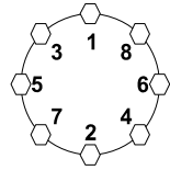
8-Lug Nuts
