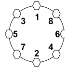
8-Lug Nuts
